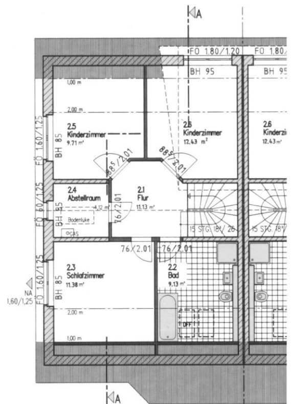
GRUNDRISS OBERGESCHOSS
