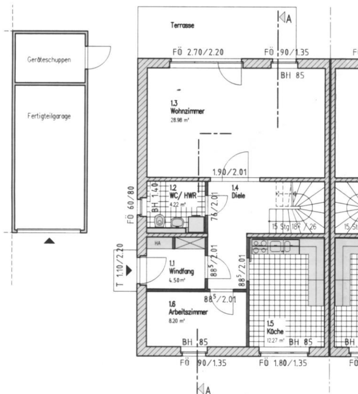
GRUNDRISS ERDGESCHOSS
